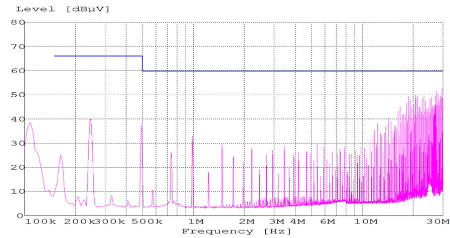
MES pre AV LIM EN 55022A V AV
