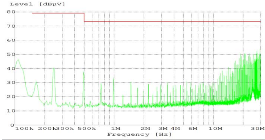
MES pre PK LIM EN 55022A V QP
