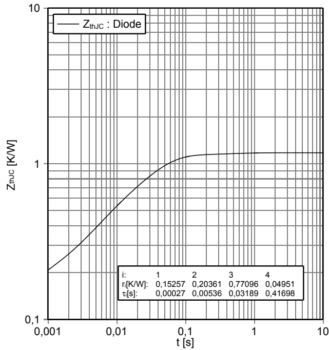
過渡熱インピーダンス Diode、リバー transient thermal impedance Diode, Reverse Z_{thJC} = f(t)
