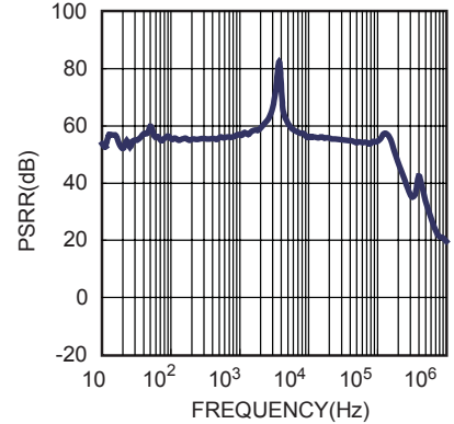
PSRR
